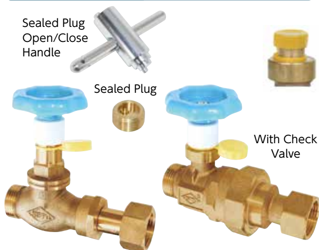
NNT Retractable Globe Valve B NNT-STE 13~25 NNT-PC Retractable Ball Valve NNT-PC-MEO 13~25
