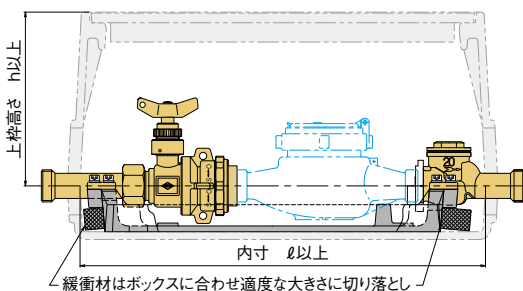
最小メータボックス寸法表
