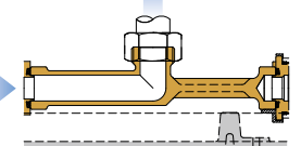
ホース接続
