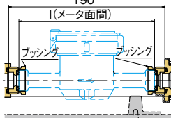
呼び径20×13L 13(面間=165)メータ使用の場合 190
