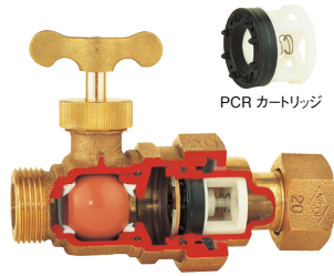
PCR-MEO 13~25
