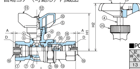
管端コア (可動形) 内蔵品
