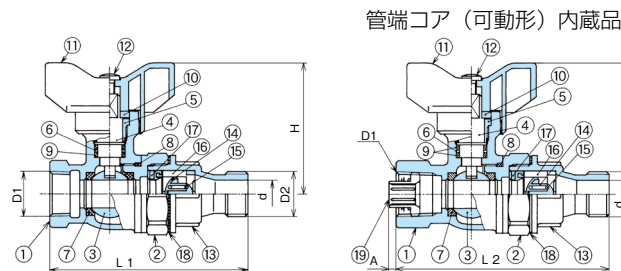
管端コア (可動形) 内蔵品
