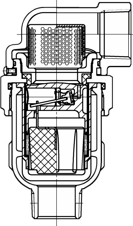
通常状態 (圧力下排気状態)
