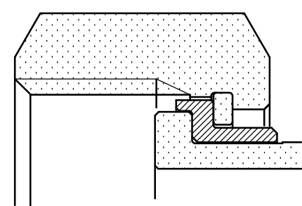
絶縁部拡大図 (2/1)
