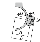
JWWA 50, 75, 100の形状
