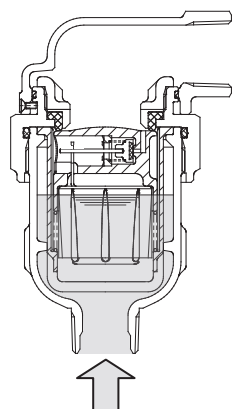
充水時(弁閉止時)
