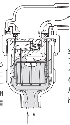
自動空気抜き時(排気時)
